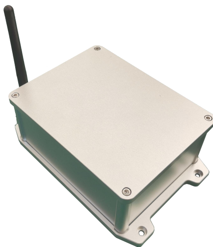
无线倾角加速度计
